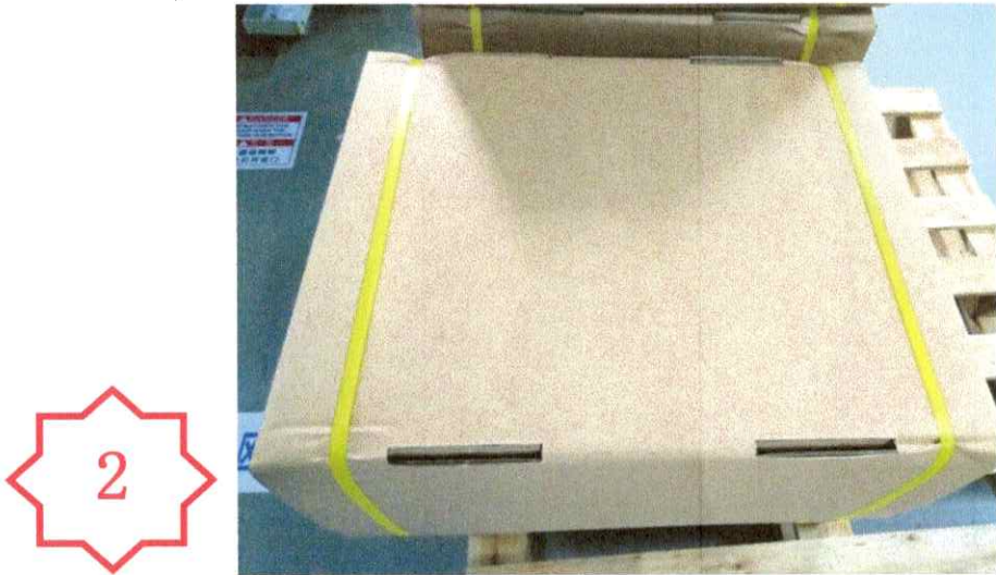
图一，一个箱子一层，一层 4 格，一格装 3 个成品，一箱共 12 个成品；将 PA03048 装入大气泡袋后再放入箱子（如图示）。
