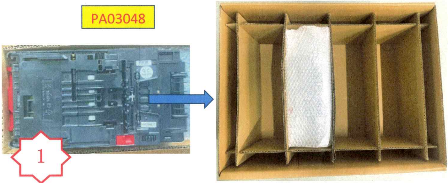
图一，一个箱子一层，一层 4 格，一格装 3 个成品，一箱共 12 个成品；将 PA03048 装入大气泡袋后再放入箱子（如图示）。
